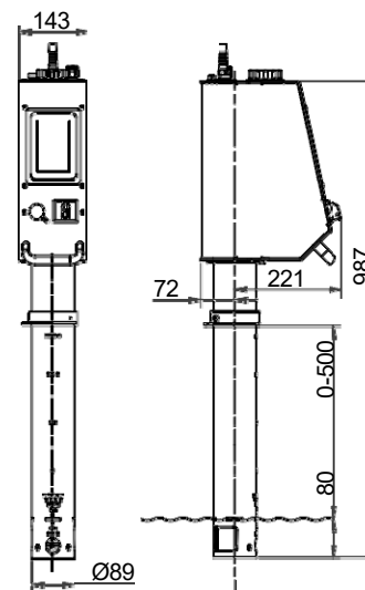
FluidWorker® 50 инсталиран на резервоар за охлаждаща течност
